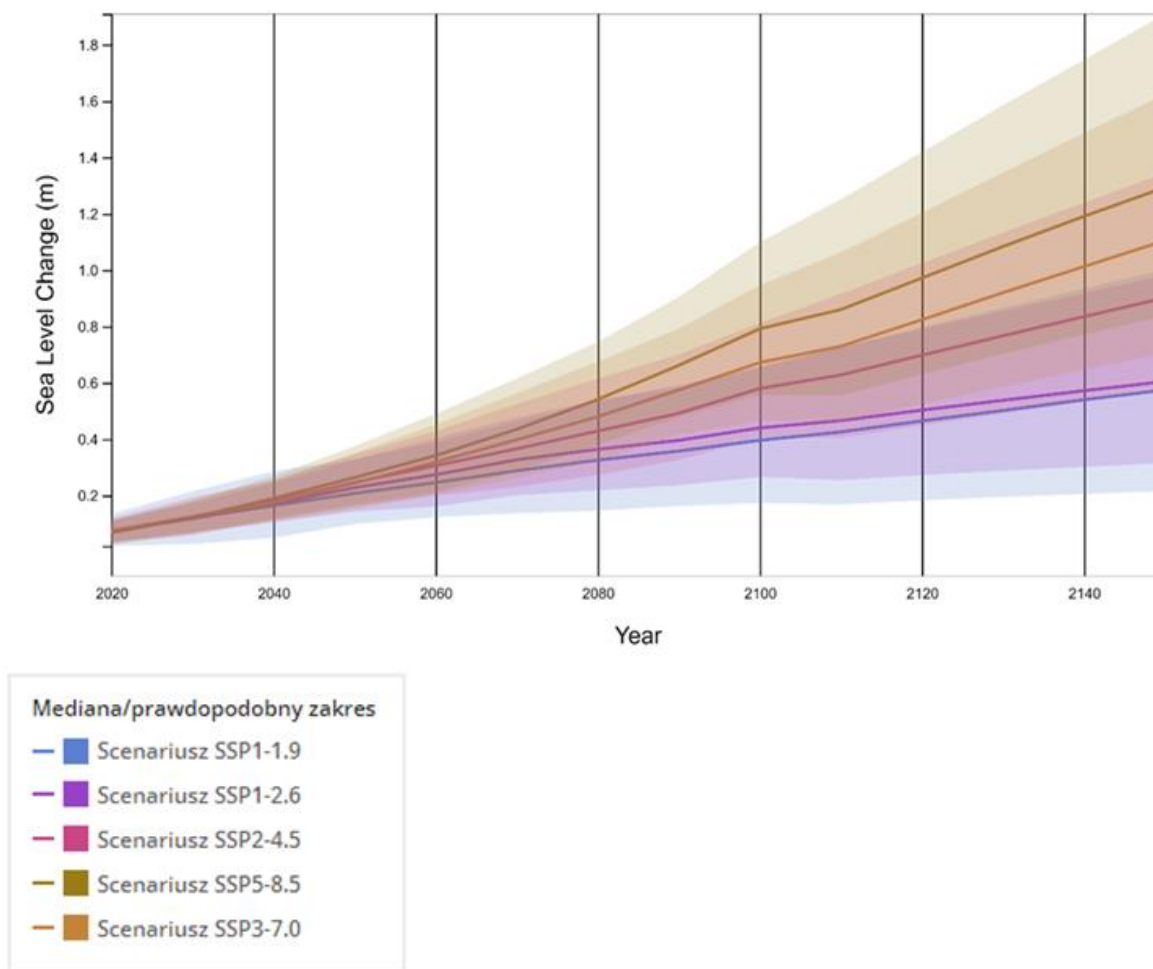
Ryc. 3 Wpływ zmian klimatu dla poszczególnych scenariuszy na średni poziom morza w Świnoujściu. Źródło: https://sealevel.nasa.gov/ipcc-ar6-sea-level-projection-tool
