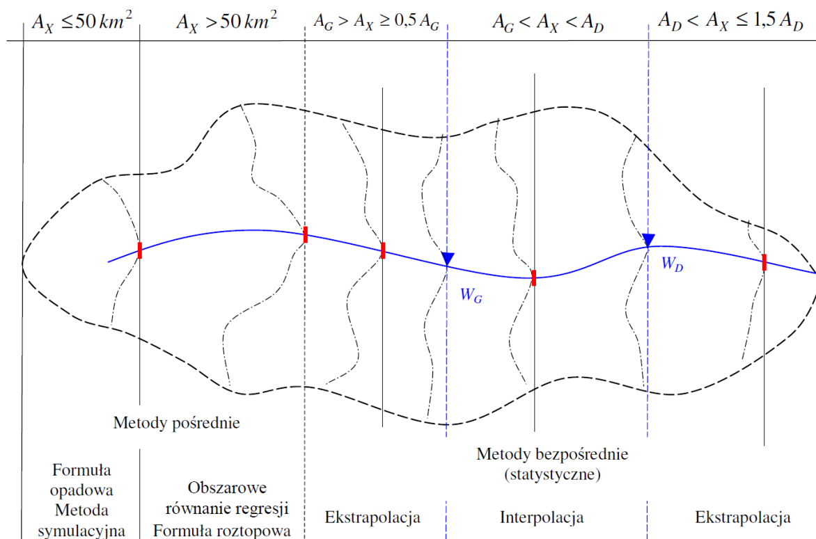
Rysunek 6. Metody obliczania przepływów maksymalnych rocznych o określonym prawdopodobieństwie przewyższenia w zlewniach kontrolowanych i niekontrolowanych (Aktualizacja metodyki..., 2017 – zmienione).
